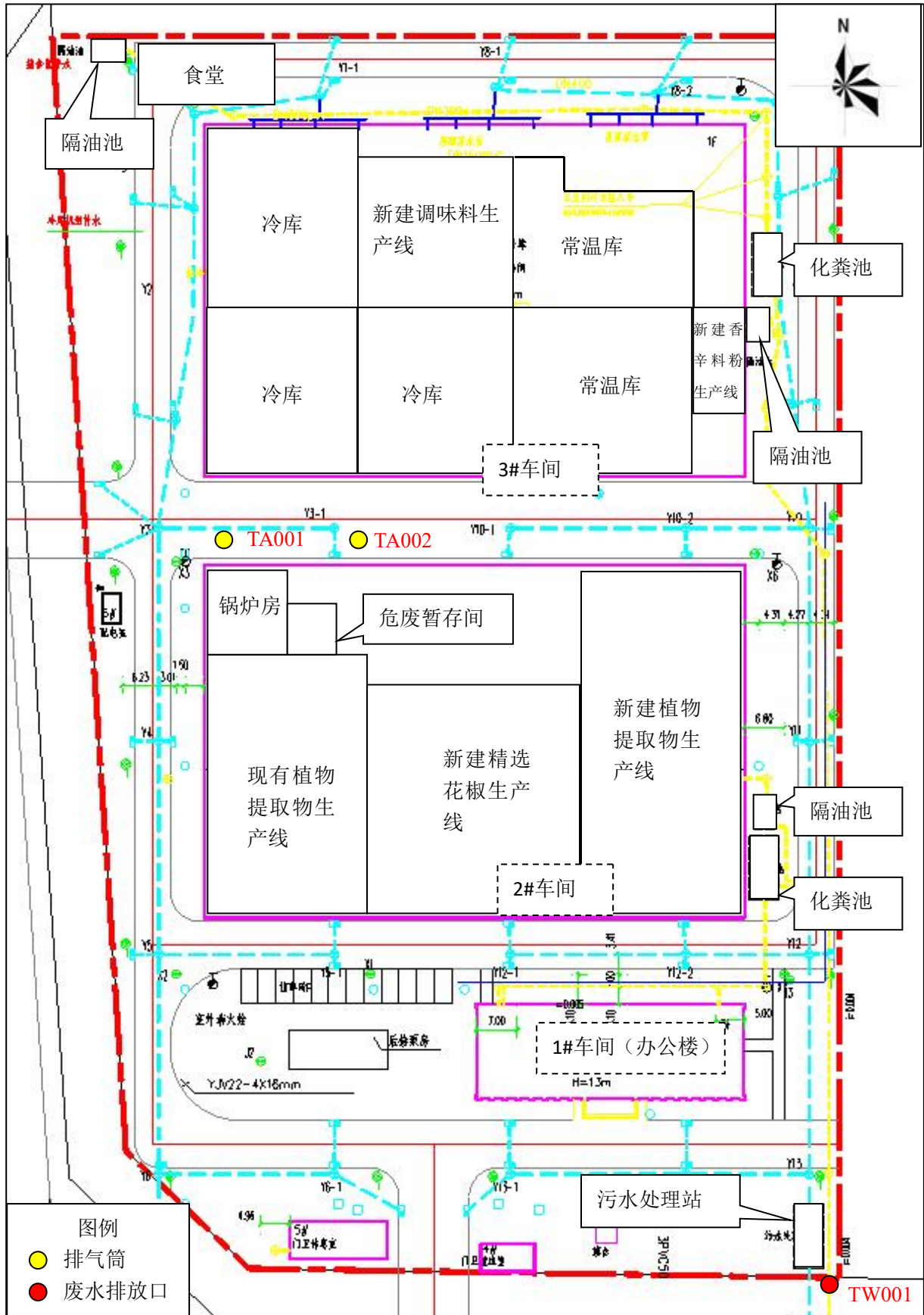
图 2 总平面布置图
