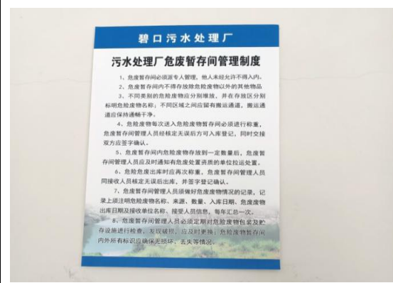
危废暂存间
