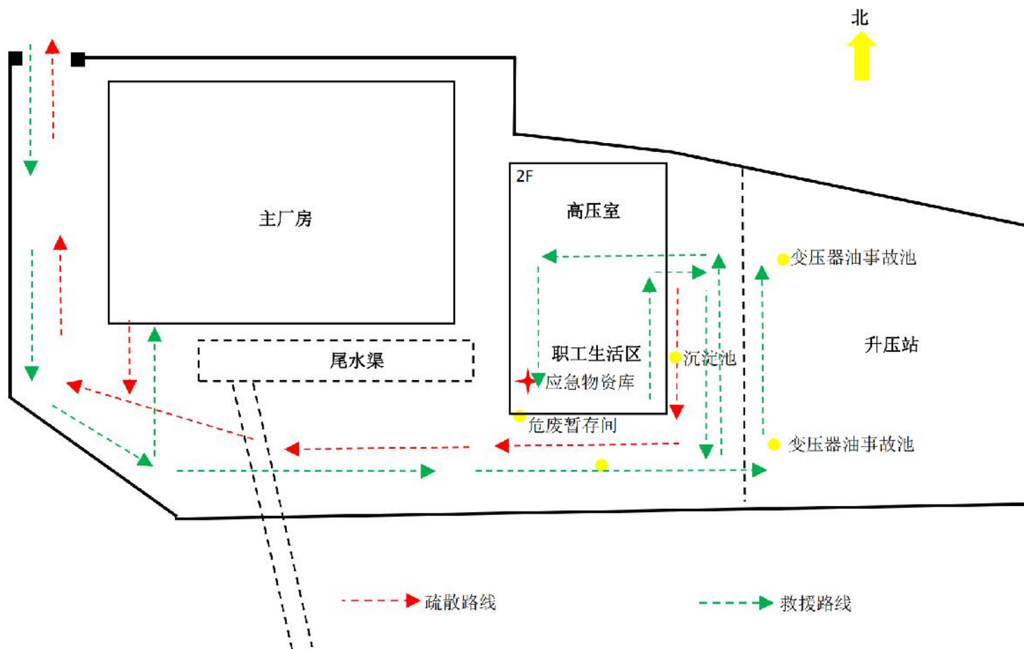
附图 4-2 建设项目平面布置、环境风险源位置及疏散线路图
