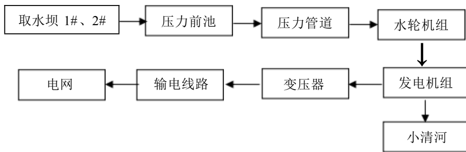
图 2.2-1 小清河二级电站生产工艺流程图
