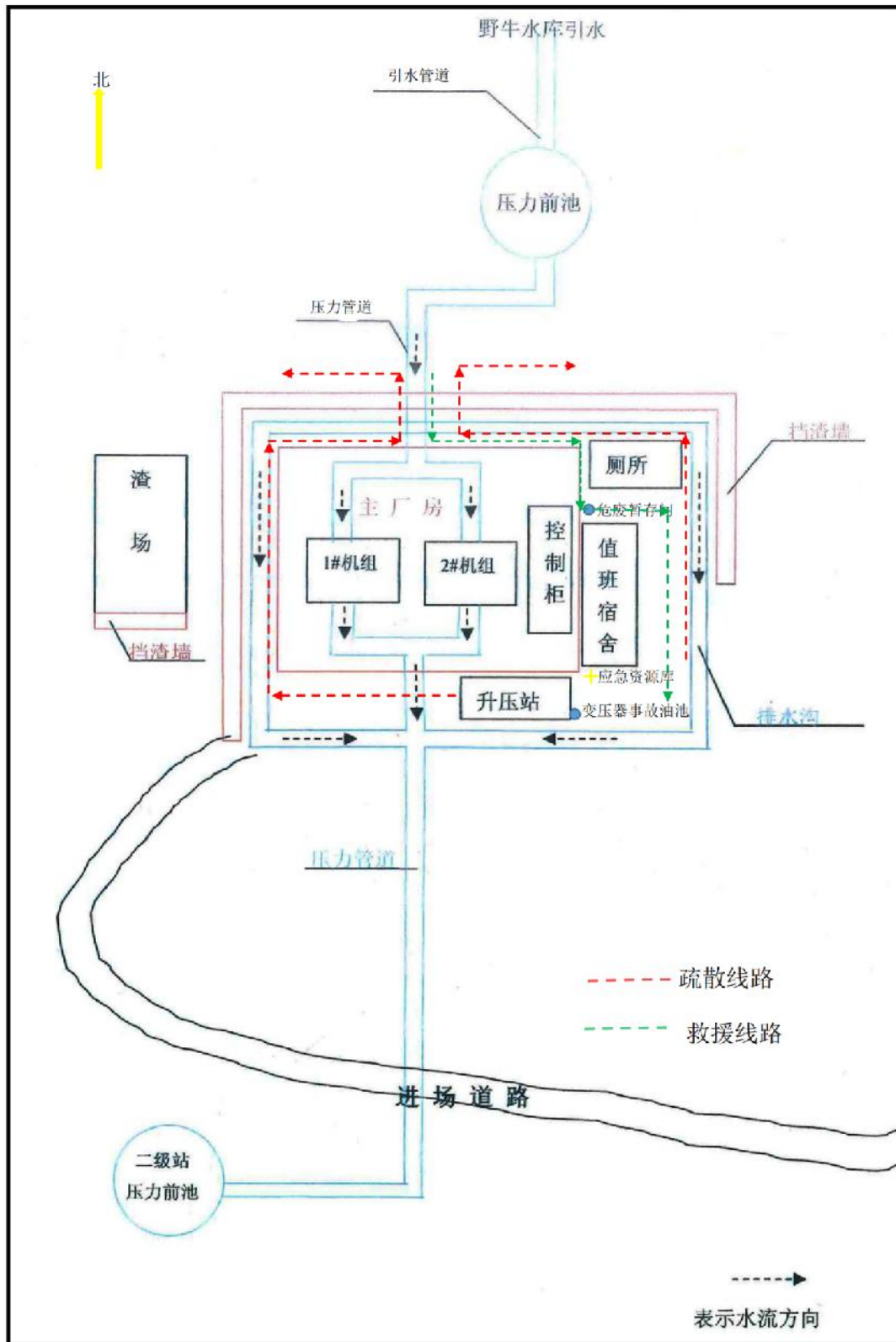
附图4 野牛一级电站厂区平面布置、环境风险源位置及疏散救援路线图
