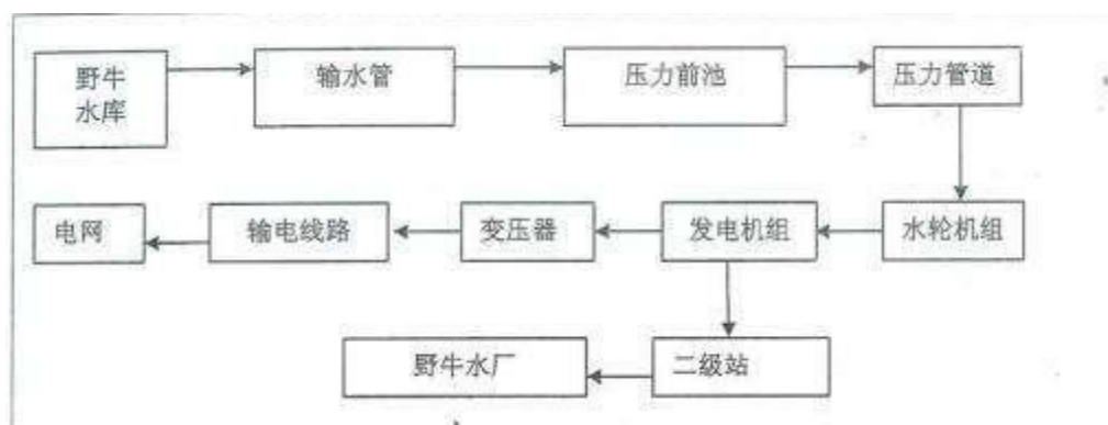
图 2.2-1 野牛一级电站生产工艺流程图
