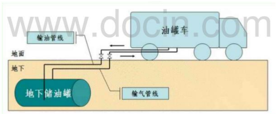
图 4-4 卸油油气回收示意图
