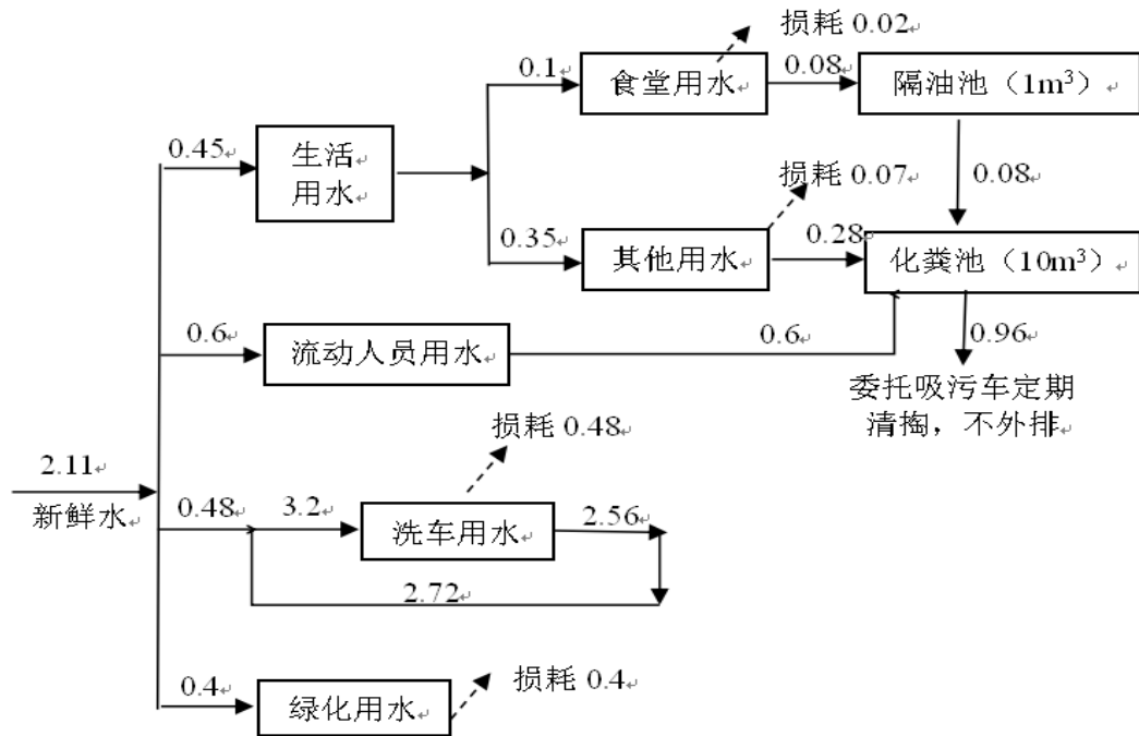
图 4-7 项目实际水平衡图 (单位: m 3 /d)
