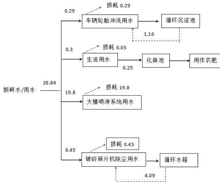
图2-1 项目水量平衡图 (m 3 /d)
