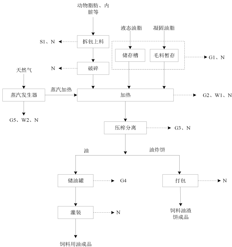
图 2-2 工艺流程及产污节点图
