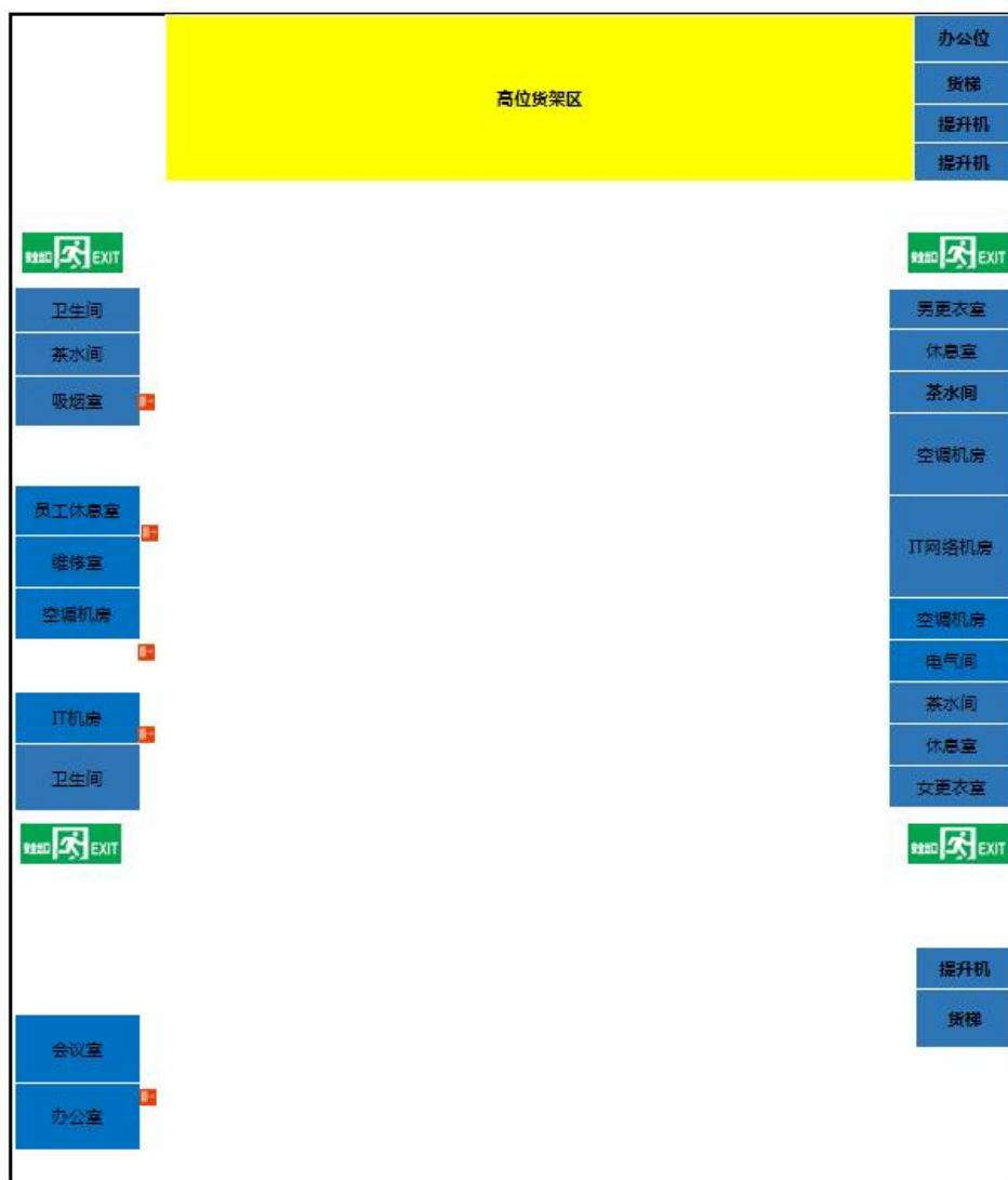
附图3-3 项目工程传动车间2F平面布置图
