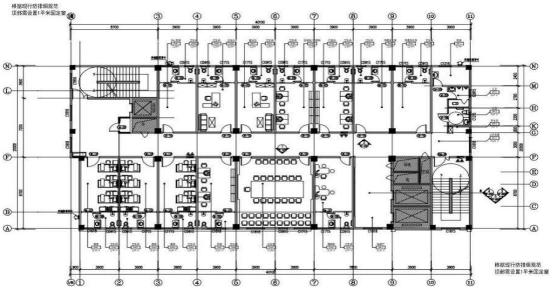
附图 2 平面布置图（综合楼 5 楼）
