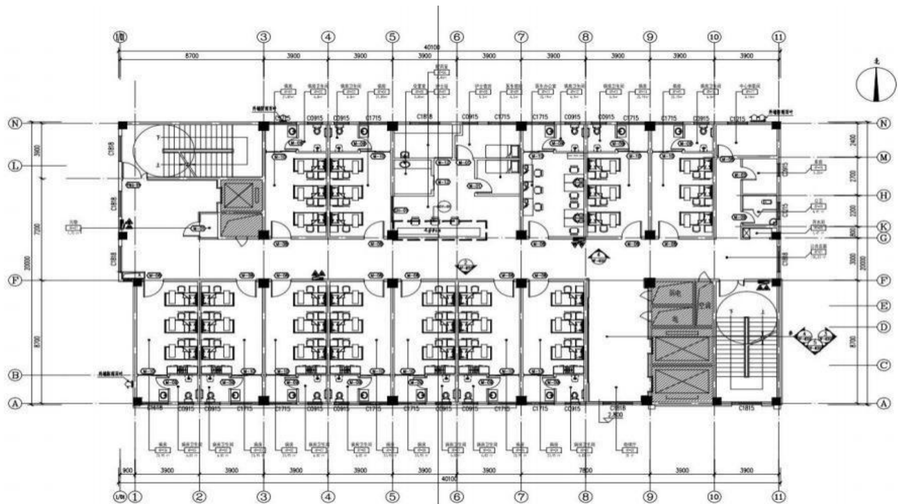
附图 2 平面布置图（综合楼 4 楼）
