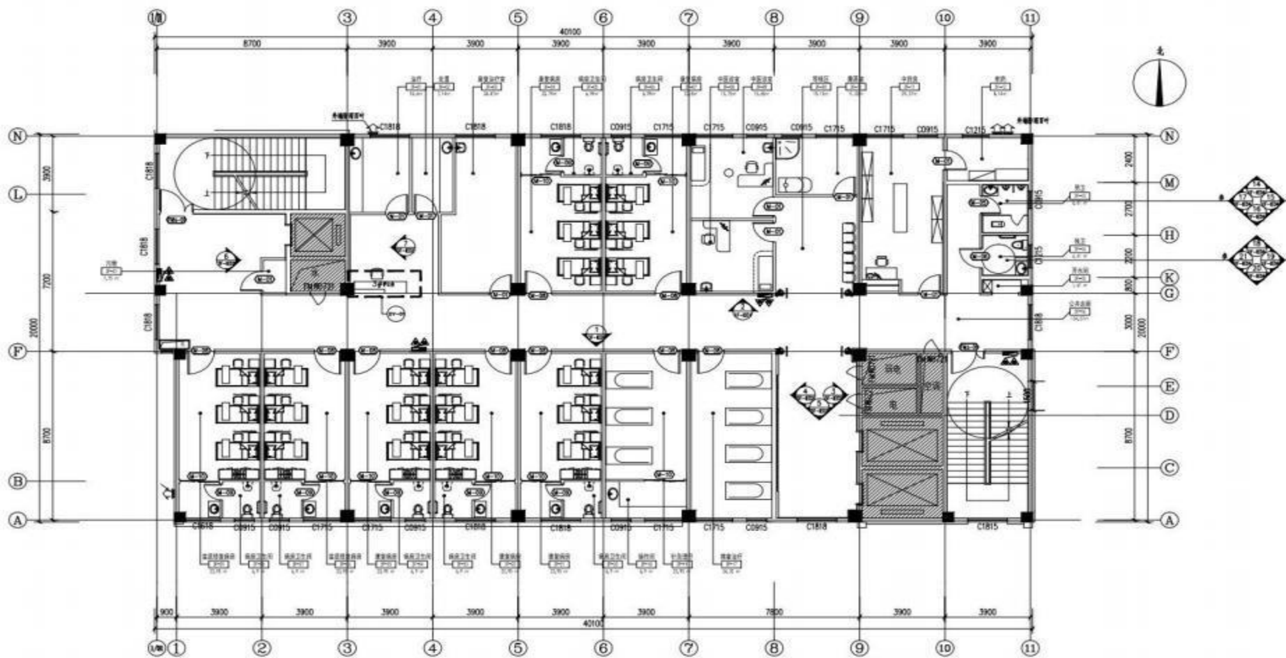
附图 2 平面布置图（综合楼 3 楼）
