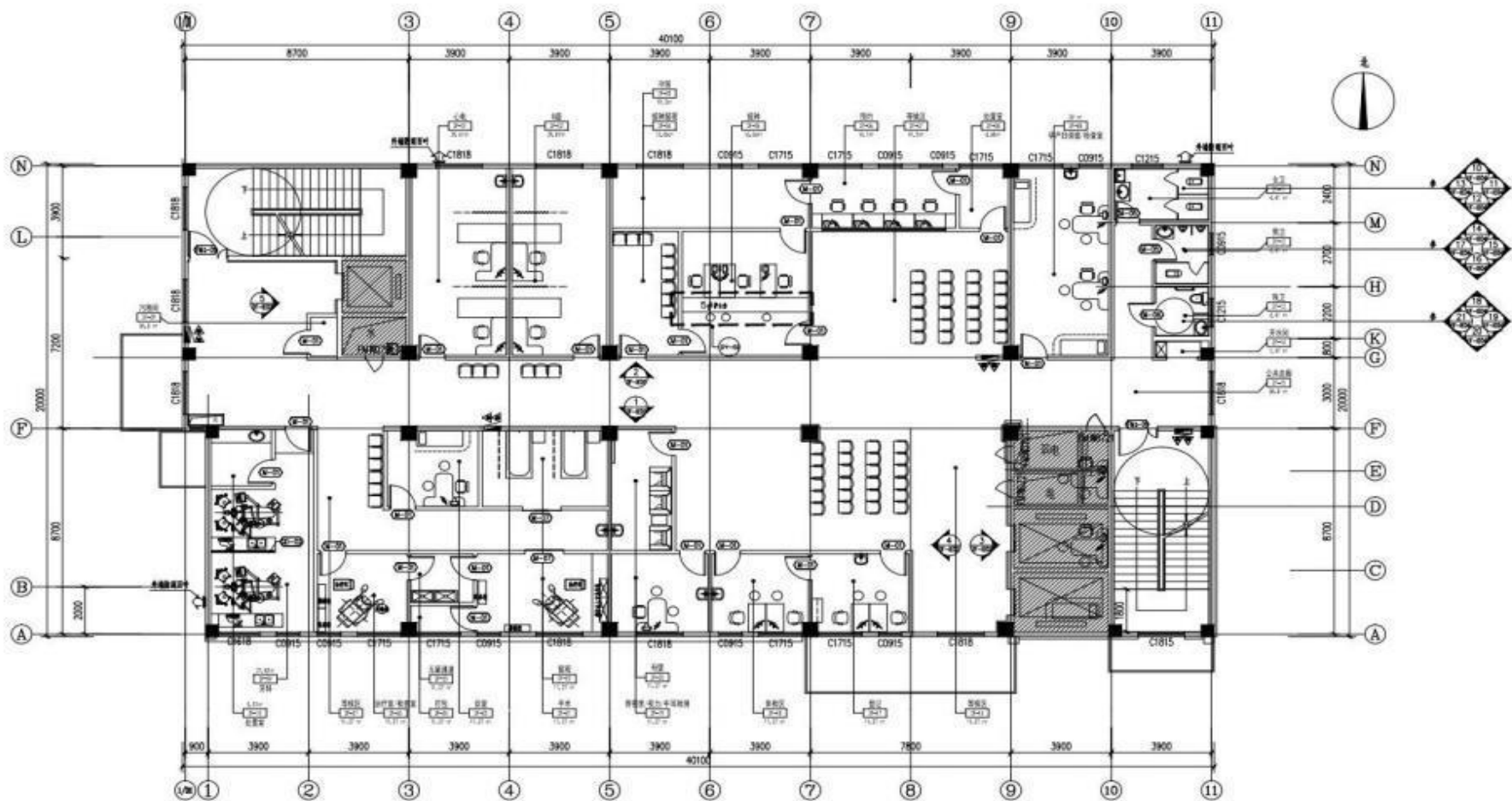
附图 2 平面布置图（综合楼 2 楼）
