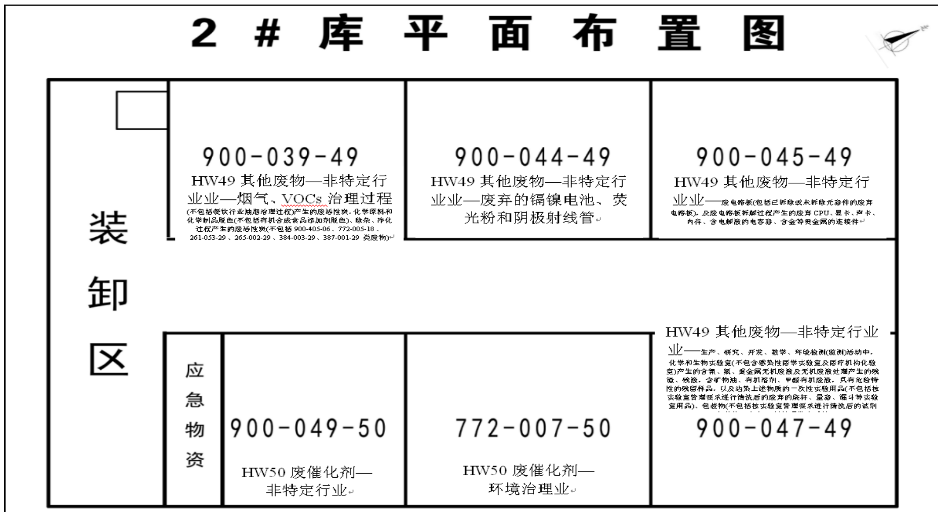
图 4 2#库—HW50 废催化剂和 HW49 其他废物贮存库平面布置示意图
