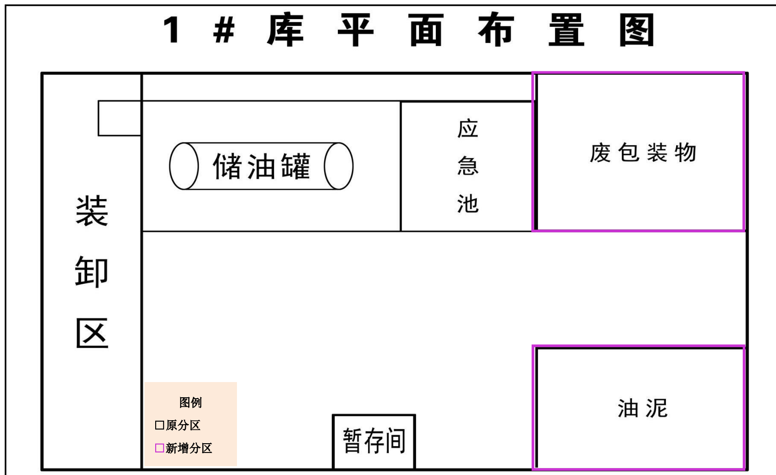
图 3 1#库—HW08 废矿物油与含矿物油废物贮存库平面布置示意图
