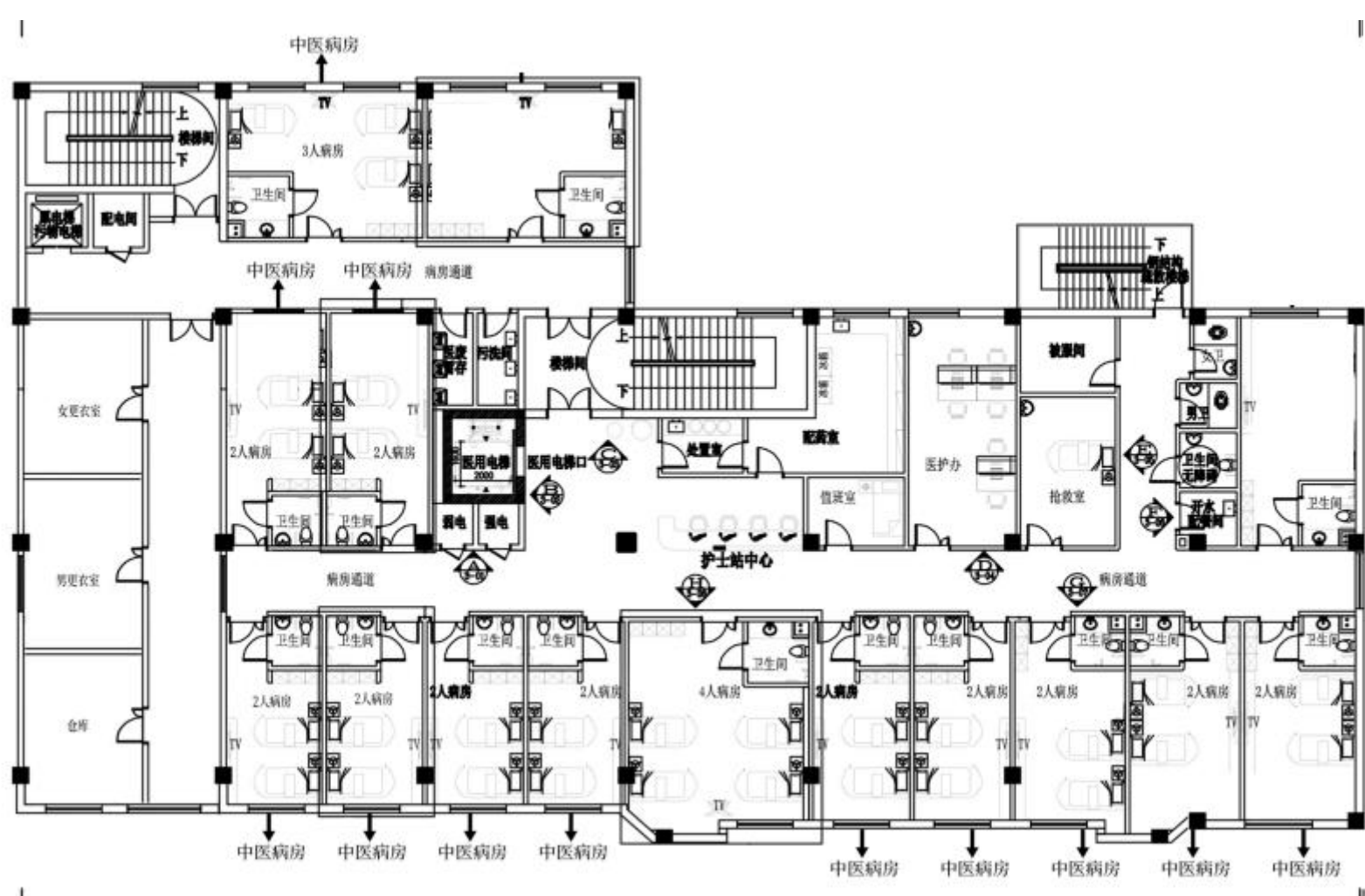
附图3-8 项目南楼三、四、五层平面布置图
