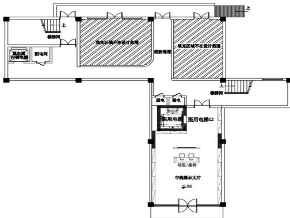
附图3-6 项目南楼一层平面布置图
