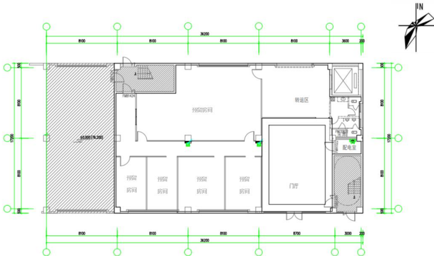
附图3-2 项目平面布置图 (1F)
