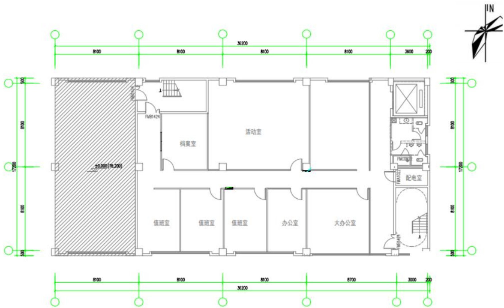
附图3-1 项目平面布置图（1F夹层）
