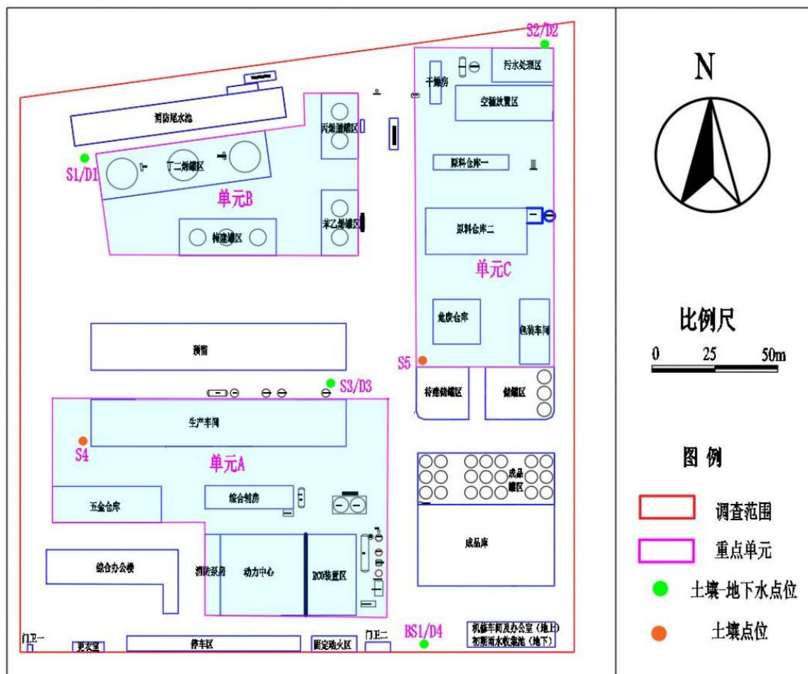
图 6.1-1 土壤和地下水布点图
