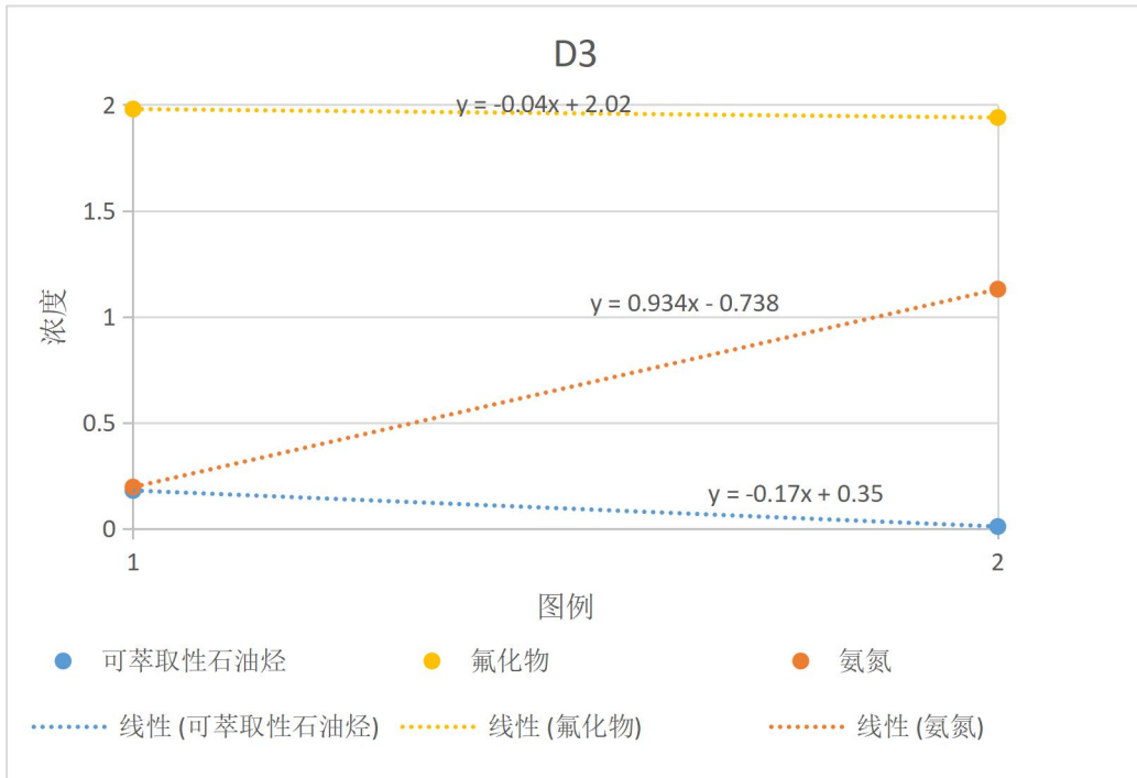
8.2-3 地下水监测井样品中 D3 监测值变化及趋势预测图
