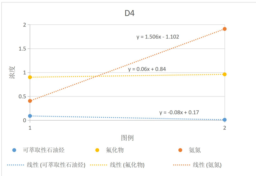
8.2-4 地下水监测井样品中 D4 监测值变化及趋势预测图
