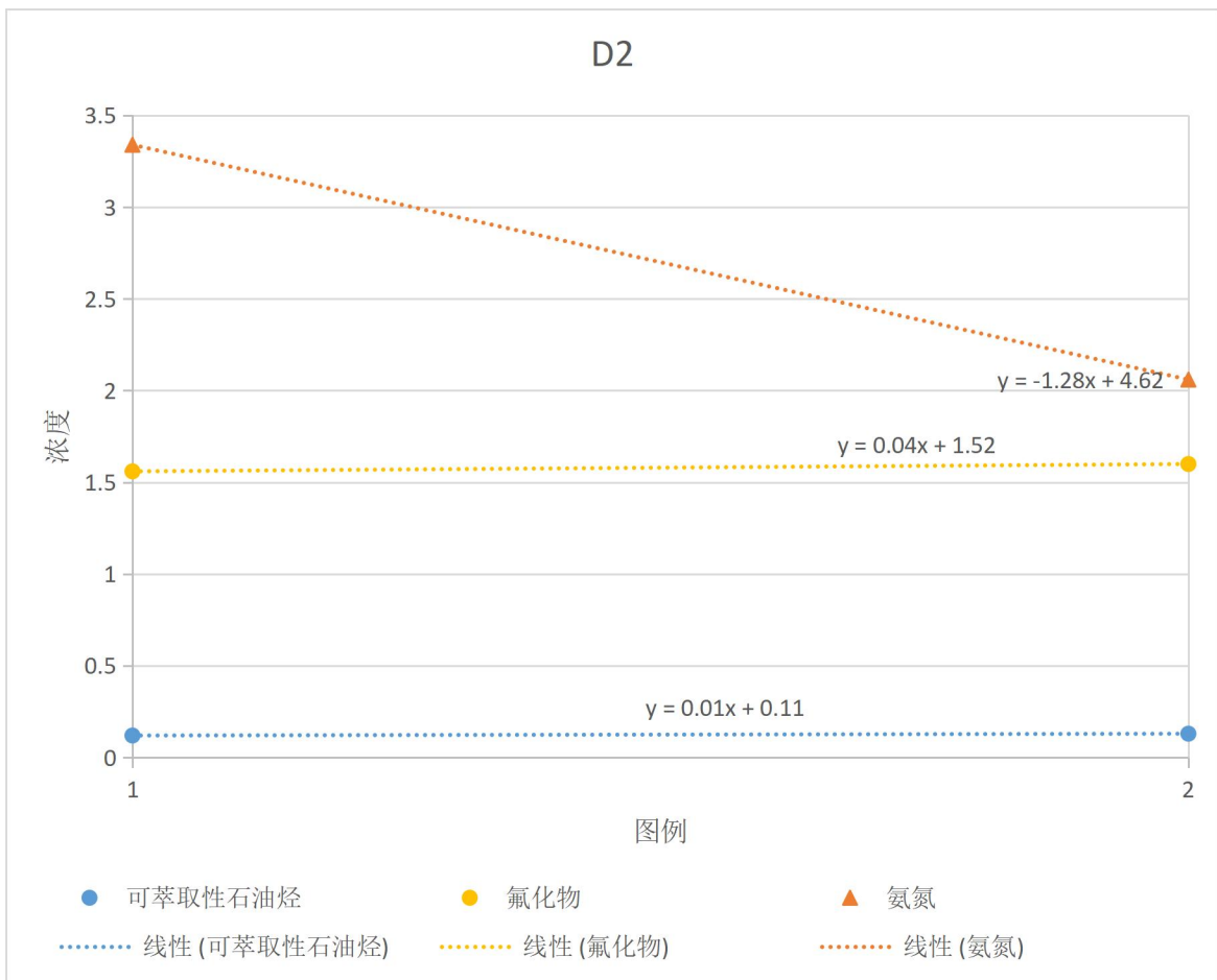
8.2-2 地下水监测井样品中 D2 监测值变化及趋势预测图
