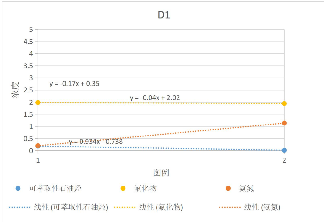
8.2-1 地下水监测井样品中 D1 监测值变化及趋势预测图
