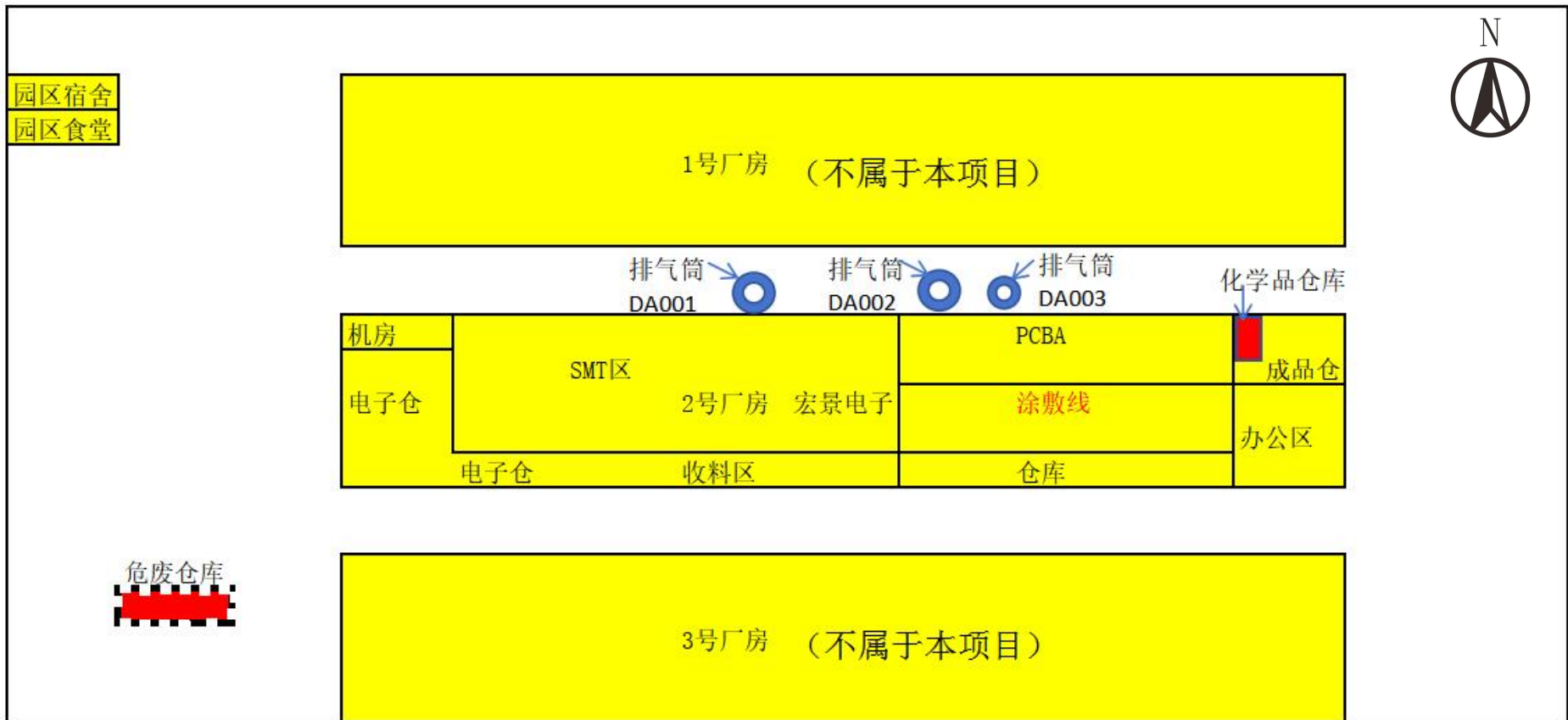
附图3-1 项目平面布置图
