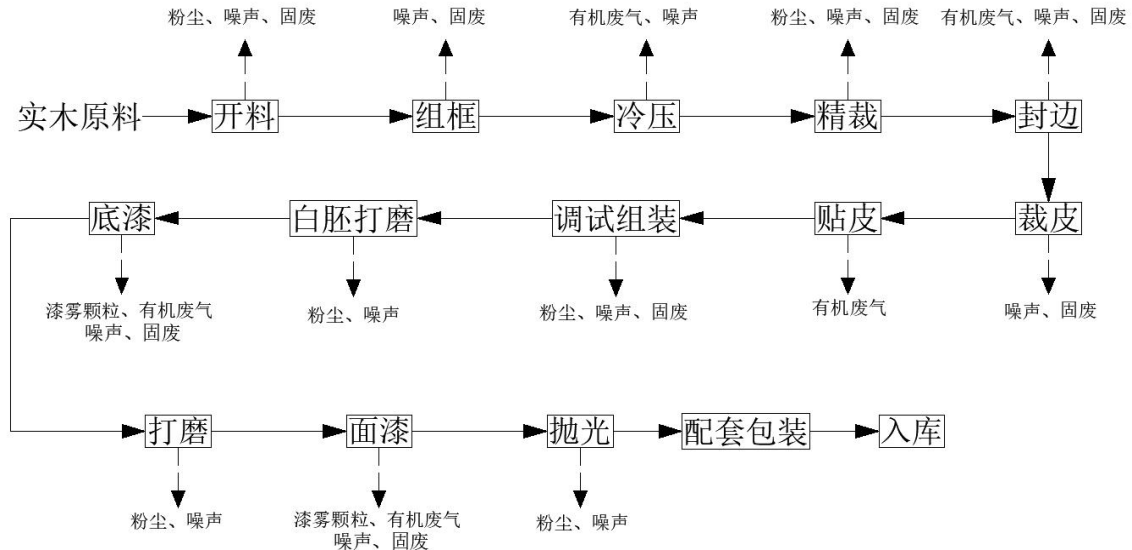
图 2.5-1 各类柜子、床和套装门生产工艺流程及产污环节示意图
