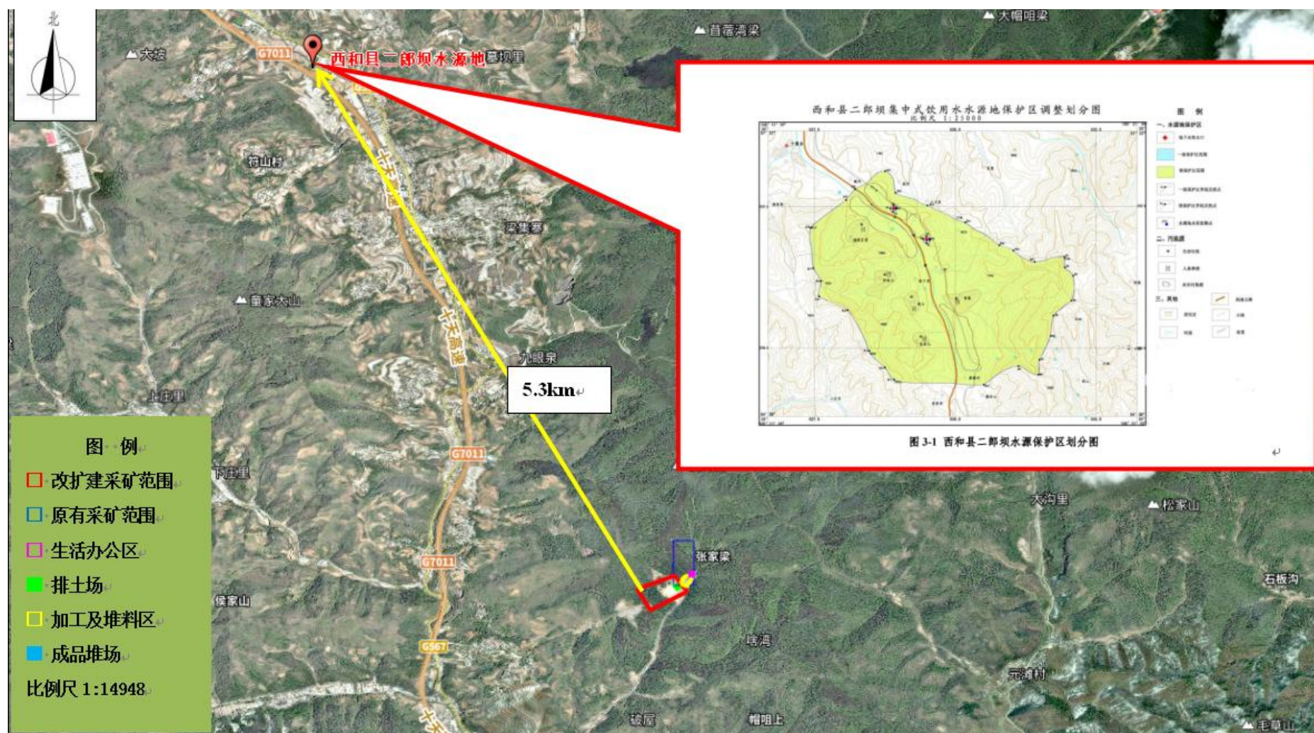
图5 项目与西和县二郎坝水源保护区位置关系图
