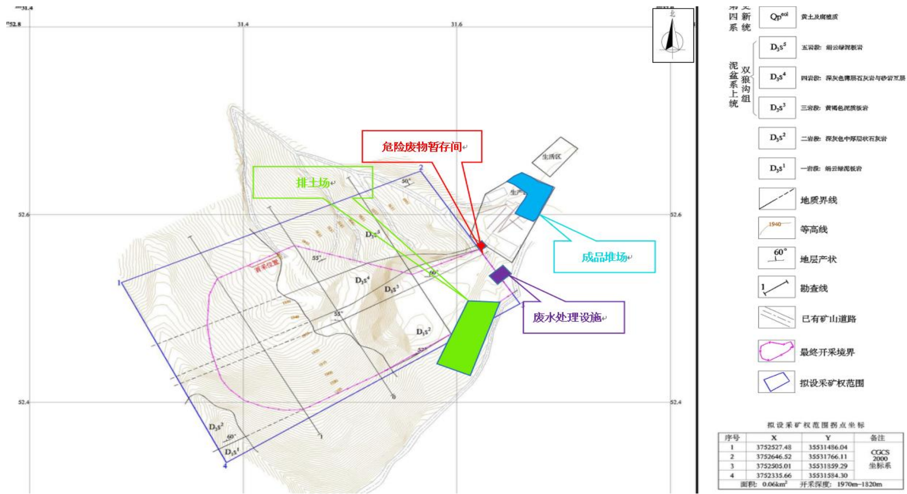
图 2 项目矿区平面布置图
