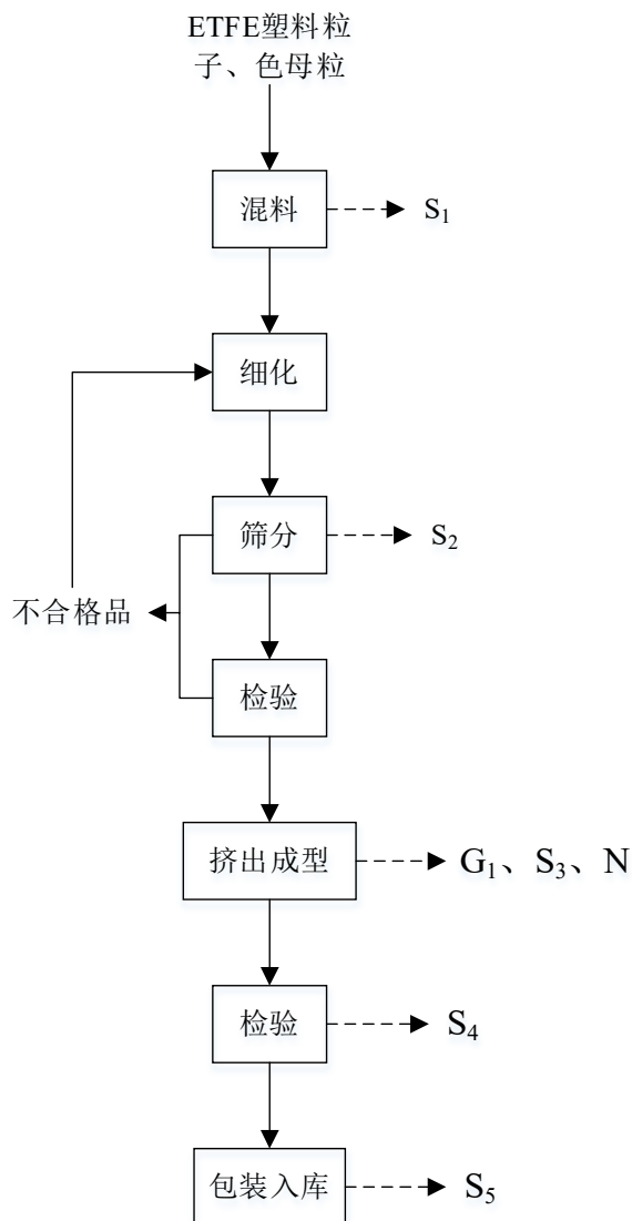
图 2-2 建设项目塑料制品生产工艺流程图
