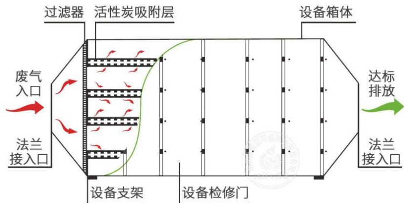
图 4-1 一般箱式活性炭内部结构示意图
