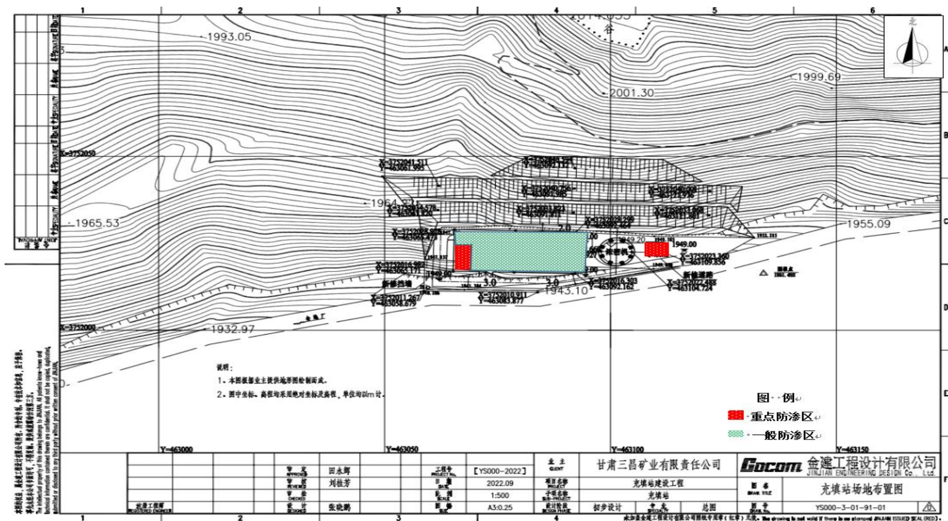
图6 项目分区防渗图
