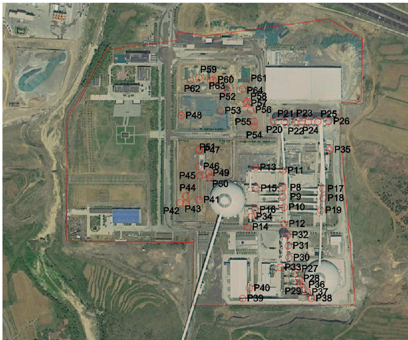
附图4 加工区排气筒点位布置图
